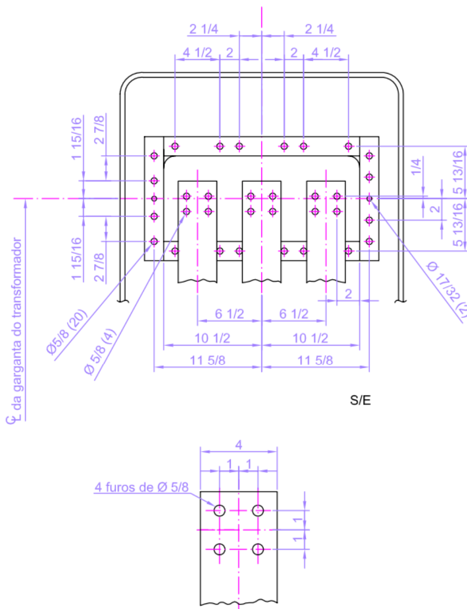
Figura 3 - Detalhes dos conectores do transformador
