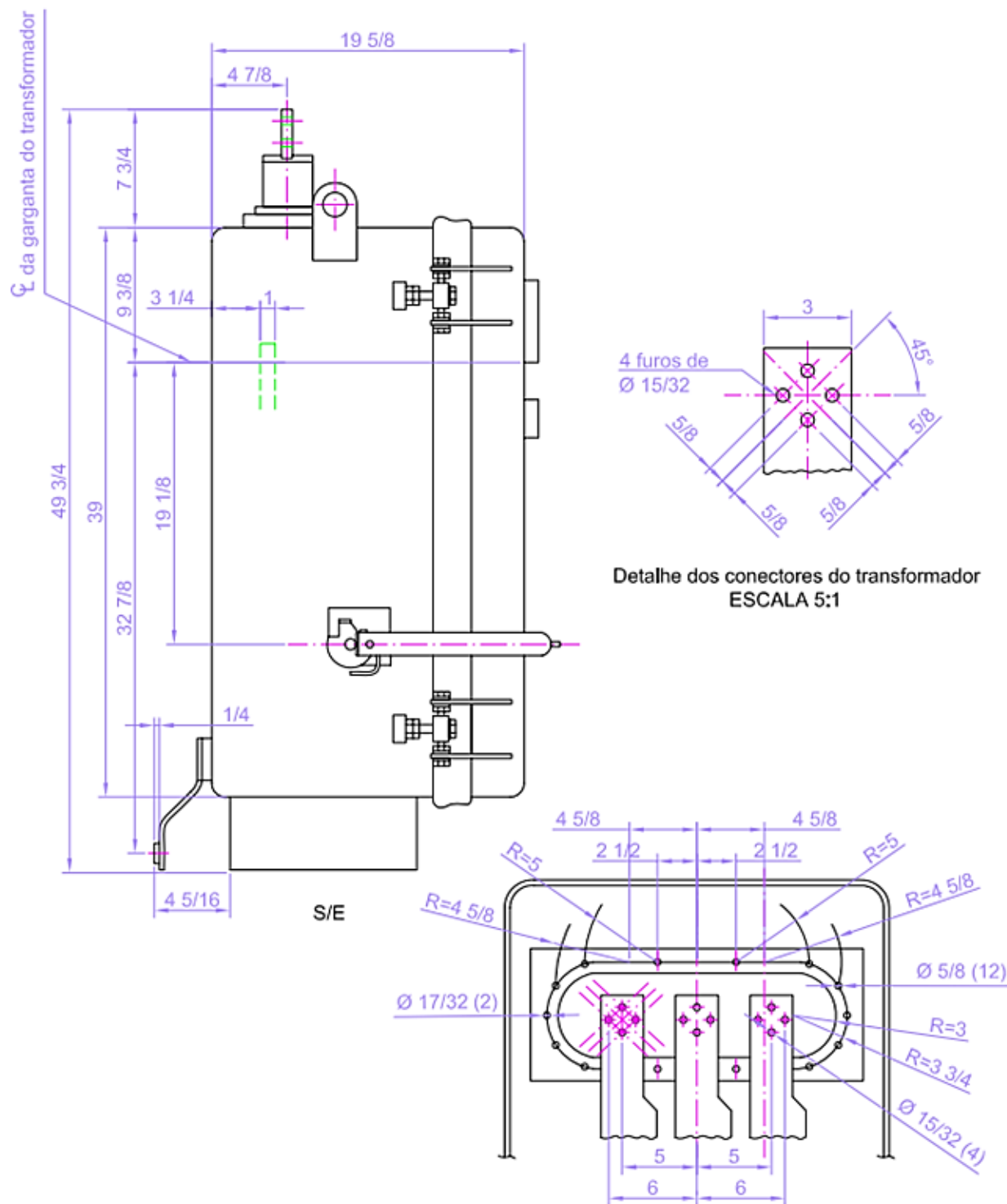
Figura 1 - Protetor do reticulado 1.200, 1.600 e 1.875A
